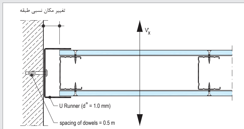
شکل ۲۱: جزئیات اطلاعات کشویی لغزان
