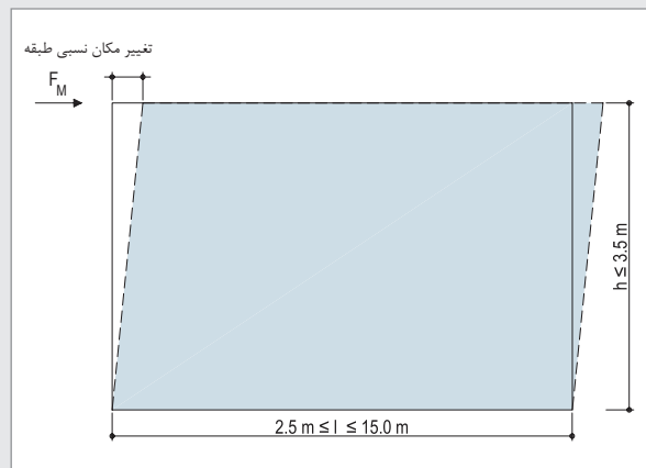
شکل ۲۰: جابه‌جایی طبقه بر اثر نیروی جنبی درون صفحه
