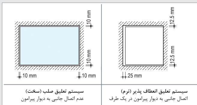
شکل ۲۵: جزئیات جداسازی سقف از دیوار پیرامون
