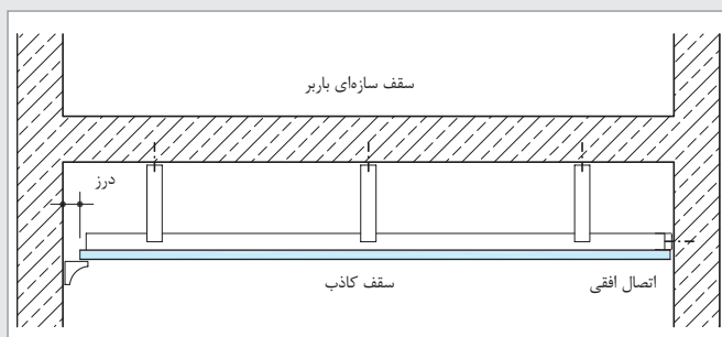
شکل ۲۶: مقطع سقف
