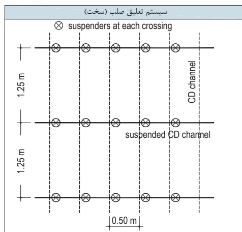
شکل ۲۳: چیدمان سیستم‌های تعلیق انعطاف پذیر و صلب
